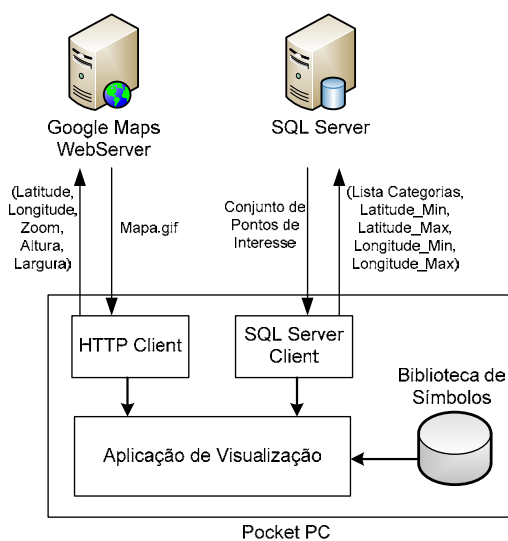
Figura 10. Arquitectura do protótipo do sistema MoViSys
