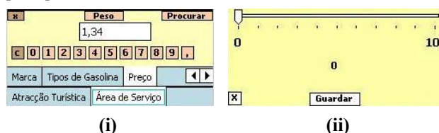
Figura 8. Mecanismo baseado em (i) text box e botões para inserir valores reais (ii) range slider para seleccionar valores ordinais
