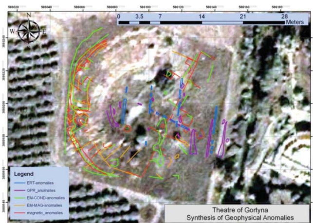
Fig. 4. Synthesis of geophysical anomalies at the Large Theatre at Gortyn. From Sarris A. – Papadopoulos N., Τεχνική έκθεση της γεωφυσικής έρευνας & χαρτογραφικής του χώρου του αρχαίου θεατρου της Γορτυνας , 2009.
