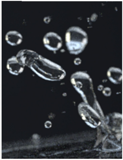
PSSMLT 0.25
