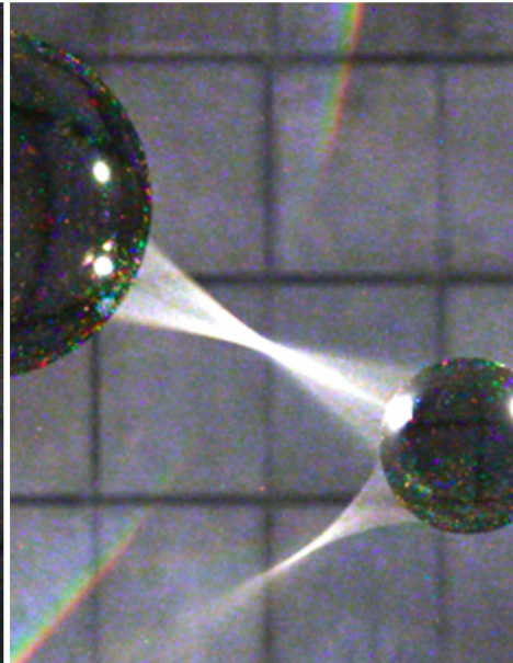
PSSMLT 0.25
