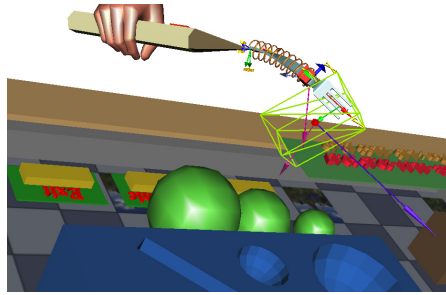
Fig. 15 Spring-fork in torsion
